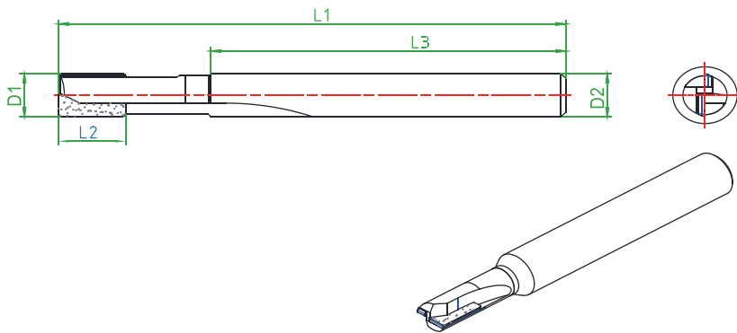
PCD End Mill--Metric
