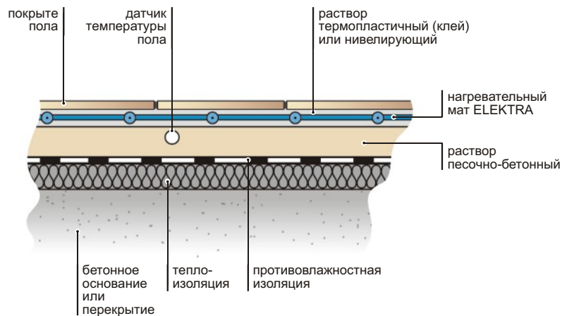
Разрез пола
