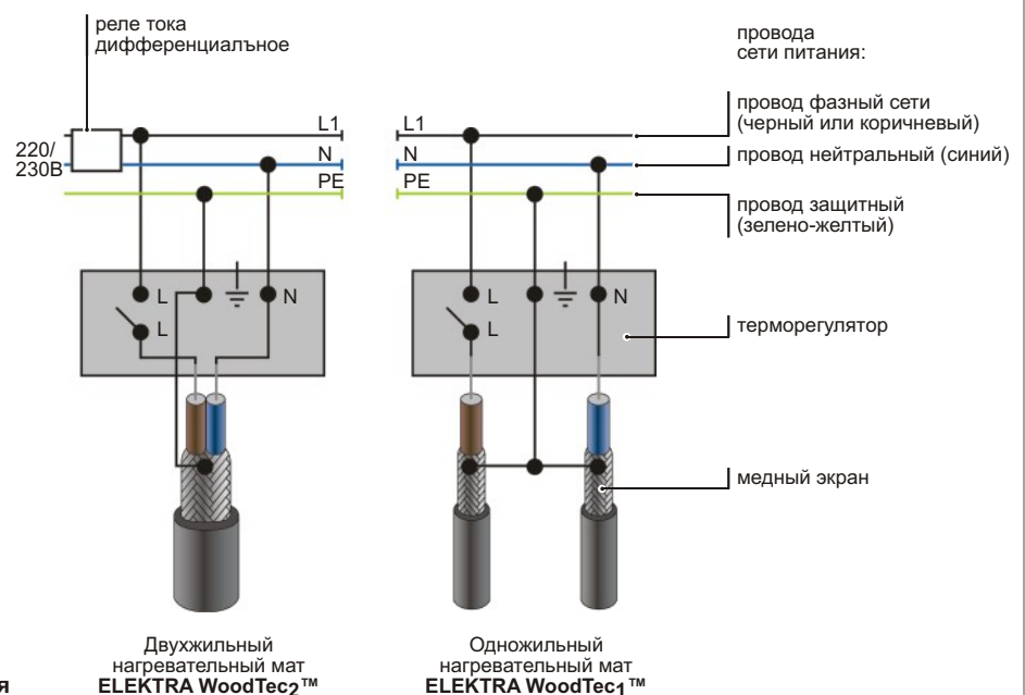
Схема подключения
