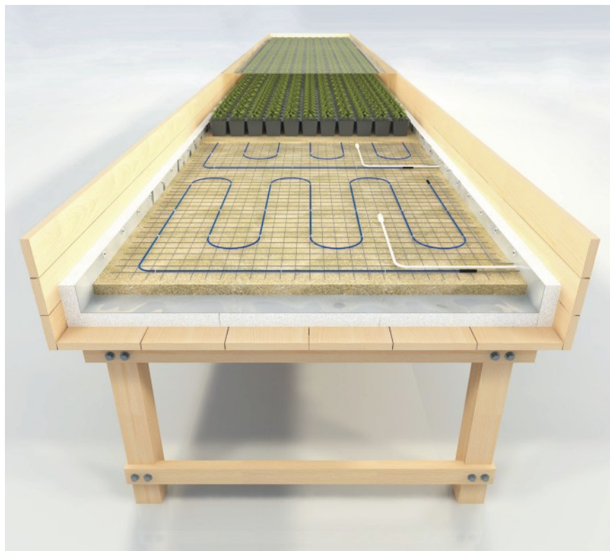
Разрез тепличного стеллажа
