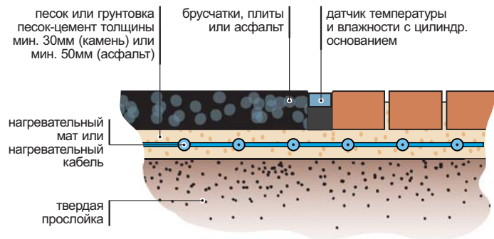
Поперечное сечение тротуара или подъездных путей, изготовленной из асфальта или брусчатки (устанавливается в слой песка)
