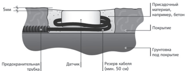
Пример монтажа датчика температуры и влажности в поверхности
