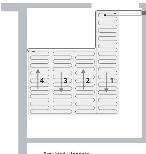
Przykład ułożenia maty grzewczej w kuchni
